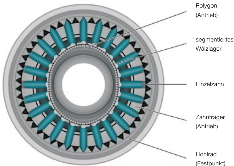
Schematischer Aufbau
